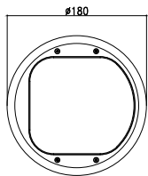
开孔尺寸: \varnothing 170 \times H138 \text{mm} \pm 1 \text{mm}
